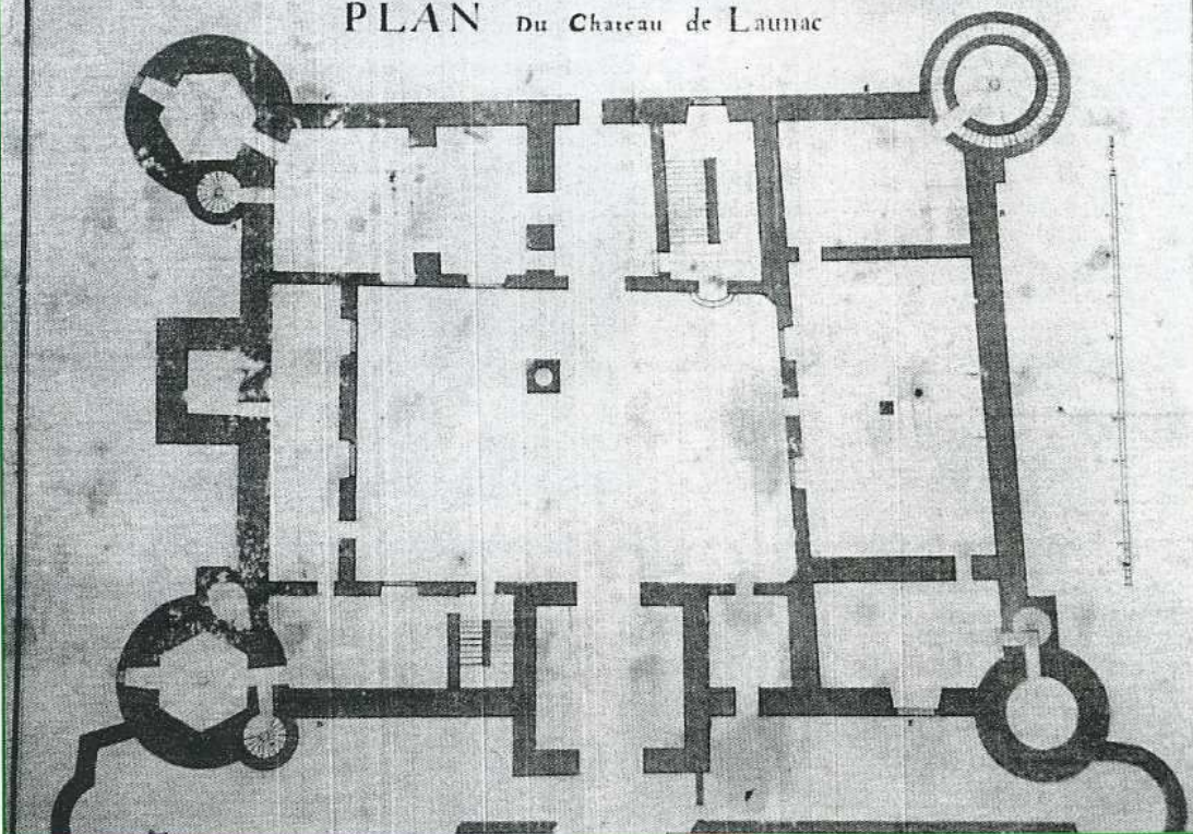
Ancien plan du château fort de Launac. En haut à droite la tour qui subsiste de nos jours. Les trois tours disparues étaient flanquées d'une tourelle abritant l'escalier.
